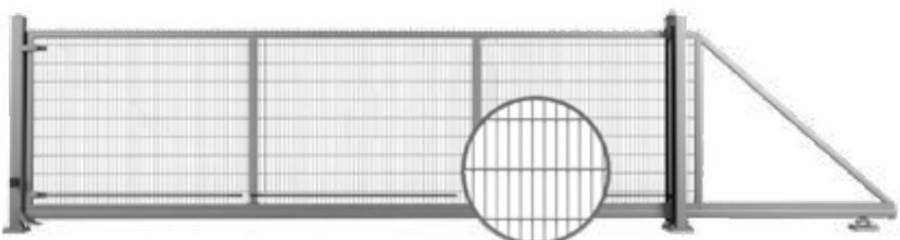
Drsna vrata z polnilom mrežaste plošče VEGA 2D Super, privarjena na konstrukcijo – pogled iz prostora.
