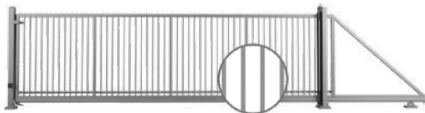
Drsna vrata s polnilom iz škatlastih profilov 25 x 25 [mm], privarjenih na konstrukcijo – pogled iz prostora.
