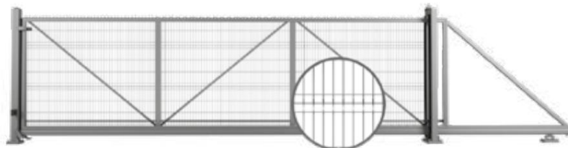
Drsna vrata s polnilom iz mrežastih plošč VEGA B privijačenih na konstrukcijo – pogled iz prostora.
